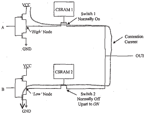
Figure 4. Drive contention due to CSRAM SEU
