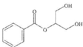
Glycerol Mono-Benzoate
