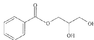
Glycerol Mono-Benzoate
