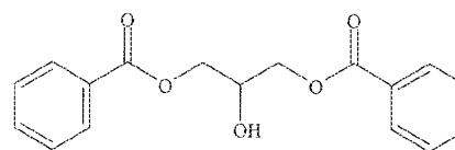
Glycerol Di-Benzoate
