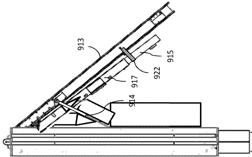
FIG. 10E
