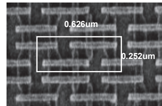
Fig.12: Top-down SEM of a 0.157 um 2 SRAM bit-cell.
