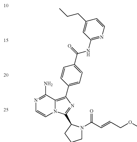
(S,E)-4-(8-Amino-3-(1-(4-methoxybut-2-en-1-yl)pyrrolidin-2-yl)imidazo[1,5-a]pyrazin-1-yl)-N-(4-propylpyridin-2-yl)benzamide
