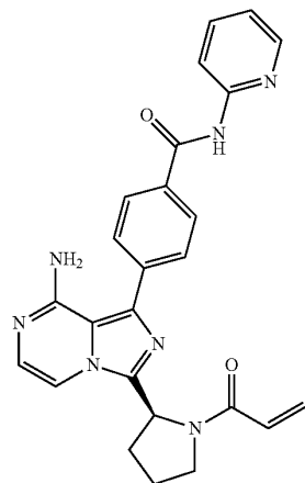
(S)-4-(3-(1-Acryloylpyrrolidin-2-yl)-8-aminoimidazo[1,5-a]pyrazin-1-yl)-N-(pyridin-2-yl)benzamide
