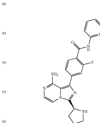
(S)-4-(8-Amino-3-(pyrrolidin-2-yl)imidazo[1,5-a] pyrazin-1-yl)-2-fluoro-N-(pyridin-2-yl)benzamide
