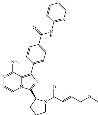
(S,E)-4-(8-amino-3-(1-(4-methoxybut-2-enoyl)pyrrolidin-2-yl)imidazo[1,5-a]pyrazin-1-yl)-N-(pyridin-2-yl)benzamide
