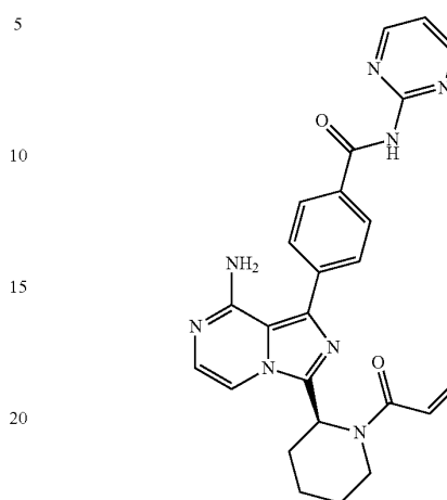
(S)-4-(3-(1-Acryloylpiperidin-2-yl)-8-aminoimidazo[1,5-a]pyrazin-1-yl)-N-(pyrimidin-2-yl)benzamide
