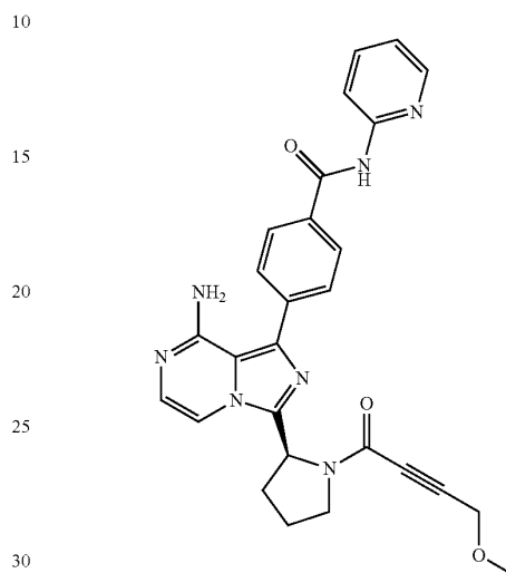
(S)-4-(8-Amino-3-(1-(4-methoxybut-2-ynoyl)pyrrolidin-2-yl)imidazo[1,5-a]pyrazin-1-yl)-N-(pyridin-2-yl)benzamide
