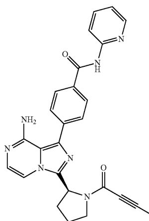
(S)-4-(8-amino-3-(1-(but-2-ynoyl)pyrrolidin-2-yl)imidazo[1,5-a]pyrazin-1-yl)-N-(pyridin-2-yl)benzamide
