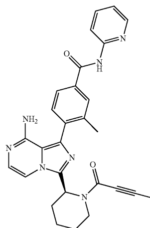
4-(8-Amino-3-((S)-piperidin-2-yl)imidazo[1,5-a]pyrazin-1-yl)-3-methyl-N-(pyridin-2-yl)benzamide
