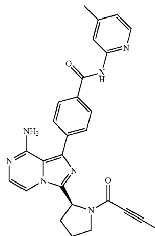
(S)-4-(8-Amino-3-(1-but-2-ynoylpyrrolidin-2-yl)imidazo[1,5-a]pyrazin-1-yl)-N-(4-methylpyridin-2-yl)benzamide
