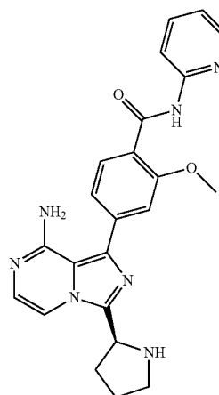
(S)-4-(8-Amino-3-(pyrrolidin-2-yl)imidazo[1,5-a]pyrazin-1-yl)-2-methoxy-N-(pyridin-2-yl)benzamide
