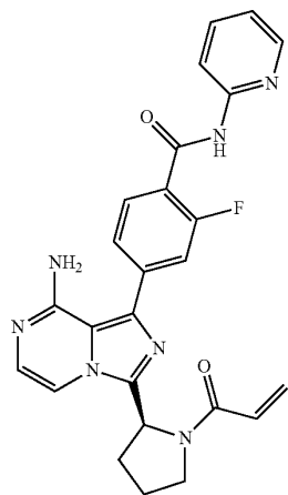
(S)-4-(3-(1-acryloylpyrrolidin-2-yl)-8-aminoimidazo[1,5-a]pyrazin-1-yl)-2-fluoro-N-(pyridin-2-yl)benzamide
