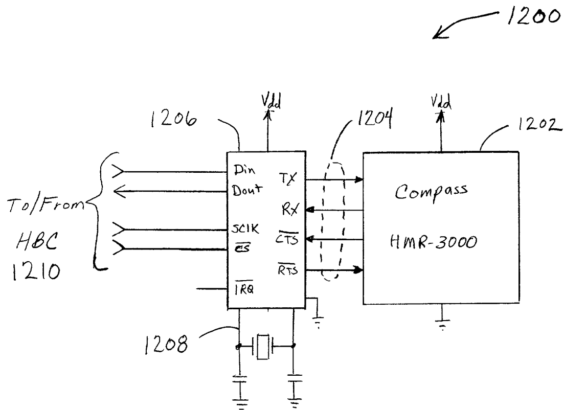
FIG. 23 Compass Module
