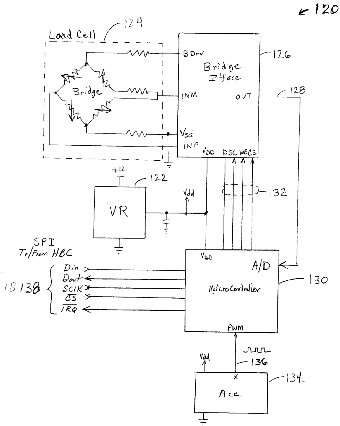
FIG. 4 Pedal Sensor Module
