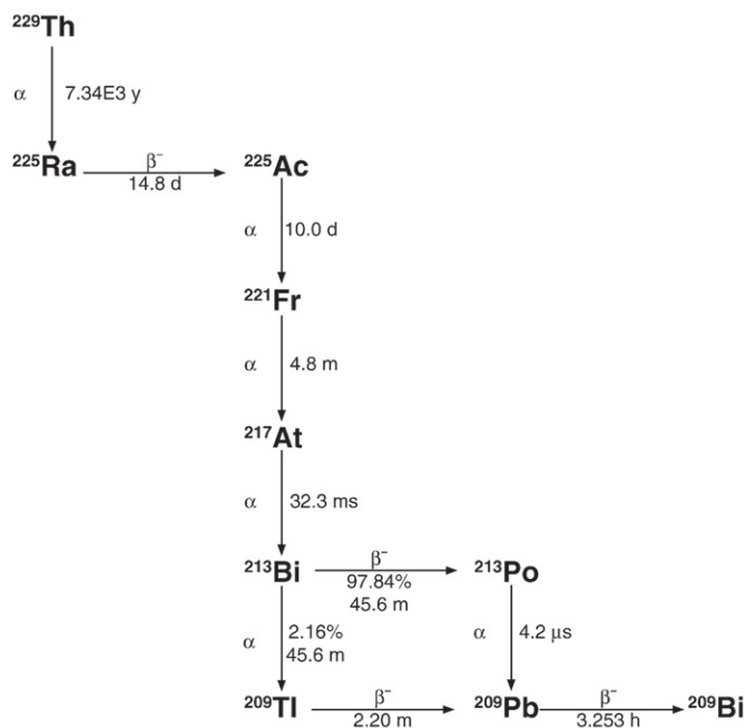
Fig. 1. The ^{229}\text{Th} decay scheme.
