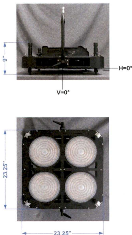
FIG. 1 LUMINAIRE
