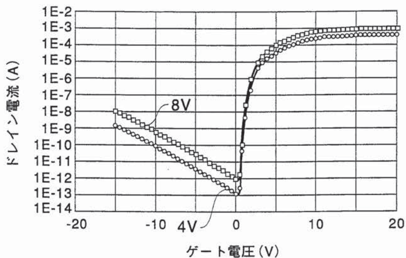
N チャネル型薄膜トランジスタの 電流電圧特性
