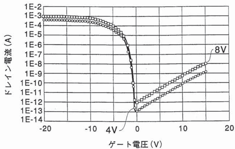
P チャネル型薄膜トランジスタの 電流電圧特性
