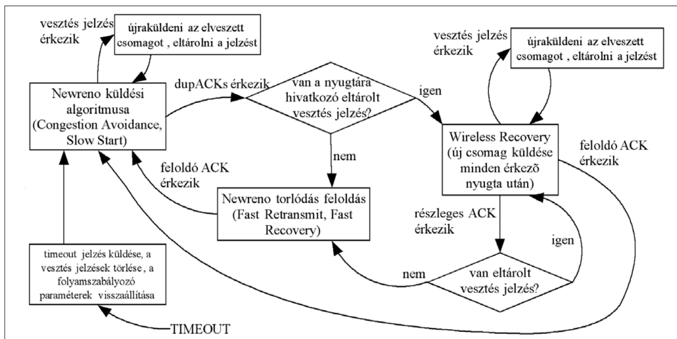
1. ábra A TCP-ELN forrás folyamatszabályozási algoritmus
