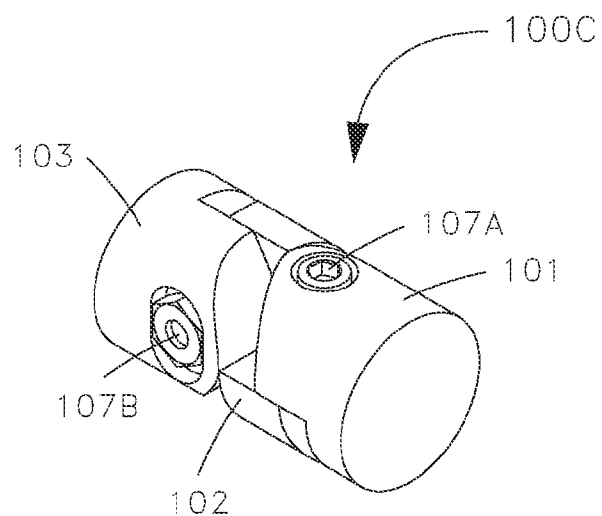
ASSEMBLED VIEW Fig. 6G
