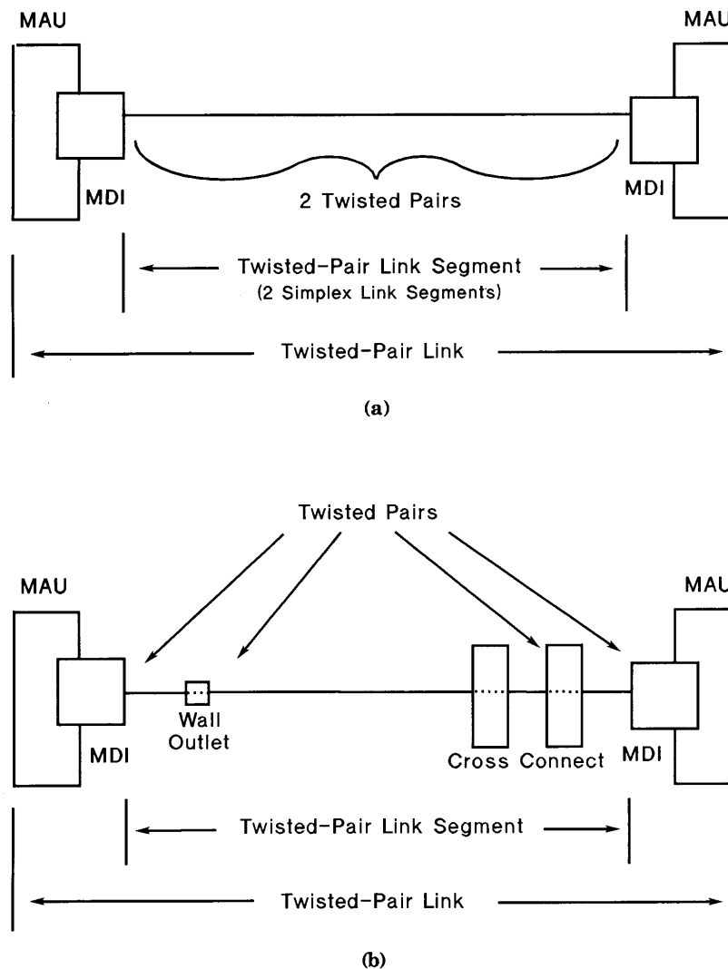
Figure 14-2—Twisted-pair link
