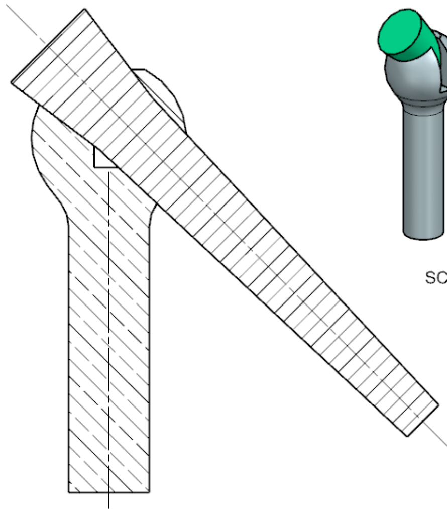
SECTION A-A
