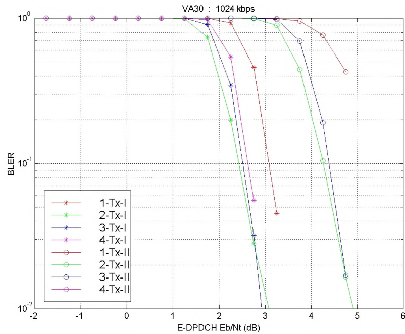
Figure A.2.2.1.12: 1024 kbps – VA30
