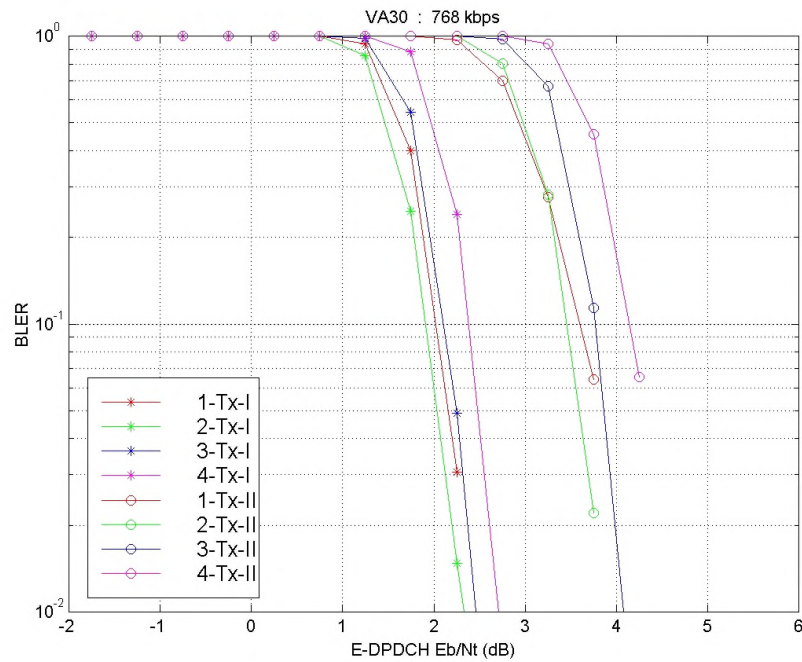
Figure A.2.2.1.10: 768 kbps – VA30
