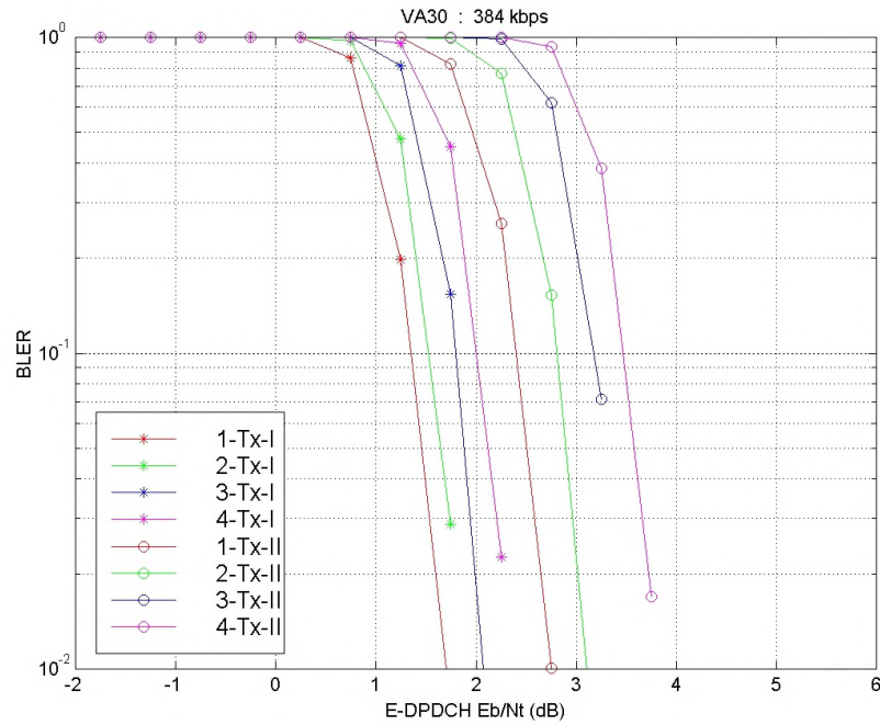
Figure A.2.2.1.7: 384 kbps – VA30
