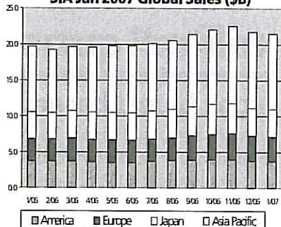
SIA Jan 2007 Global Sales ($B)
