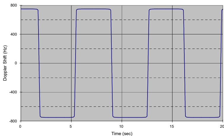
Figure B.3-1: Doppler shift trajectory
