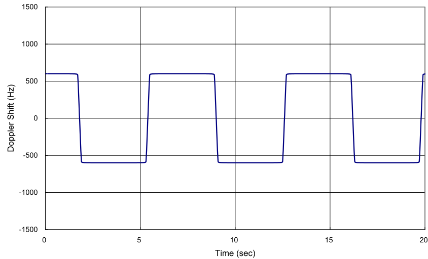
Figure B.3: Doppler shift trajectory
