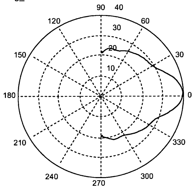
polar_0deg_2500Hz
