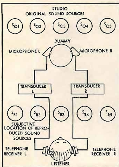
Fig. 2. Binaural.
