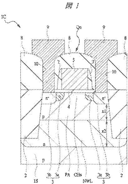
1S:半導体基板 NWL:nウエル Qp:nチャネル型のMIS・FET PA:p型の半導体領域
