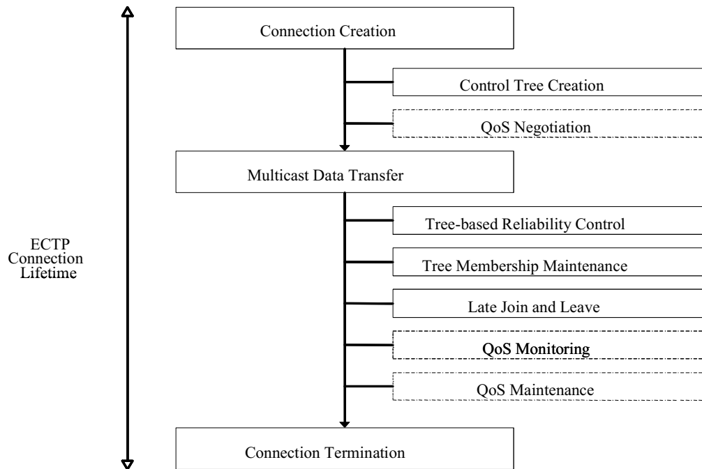
Figure 31: ITU ECTP QoS model
