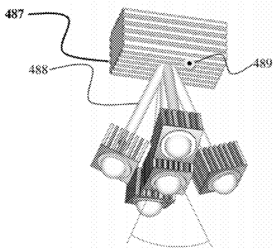
FIG. 25A
