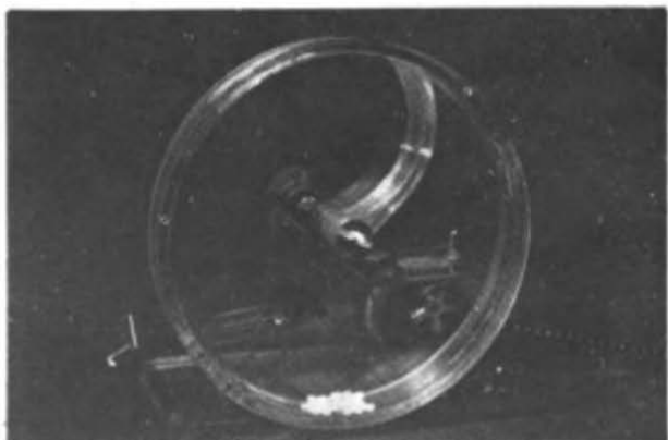
Fig 37. The Roche friabilator (courtesy, Hoffmann-LaRoche).
