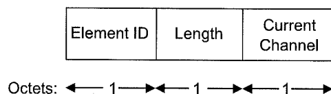
Figure 38—DS Parameter Set element format
