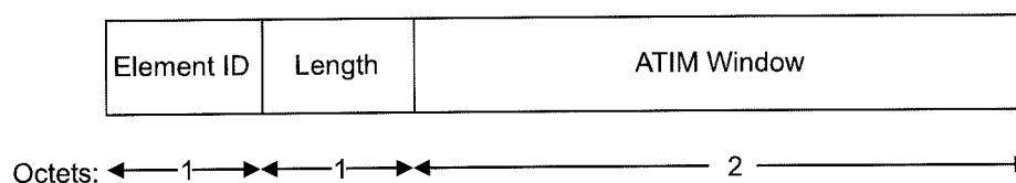
Figure 41—IBSS Parameter Set element format
