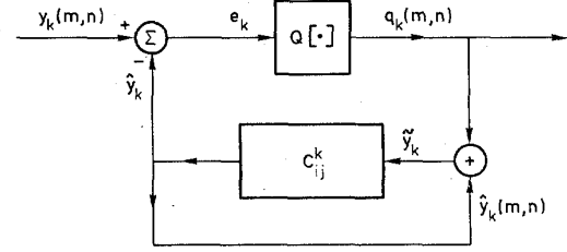
Fig. 10. DPCM for subband k .
