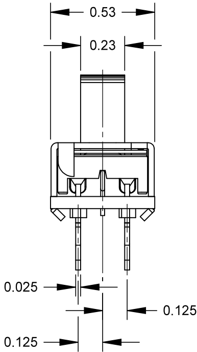
46313LDRX SHOWN
