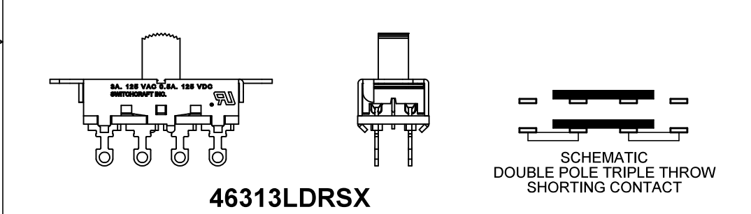
46313LDRX
