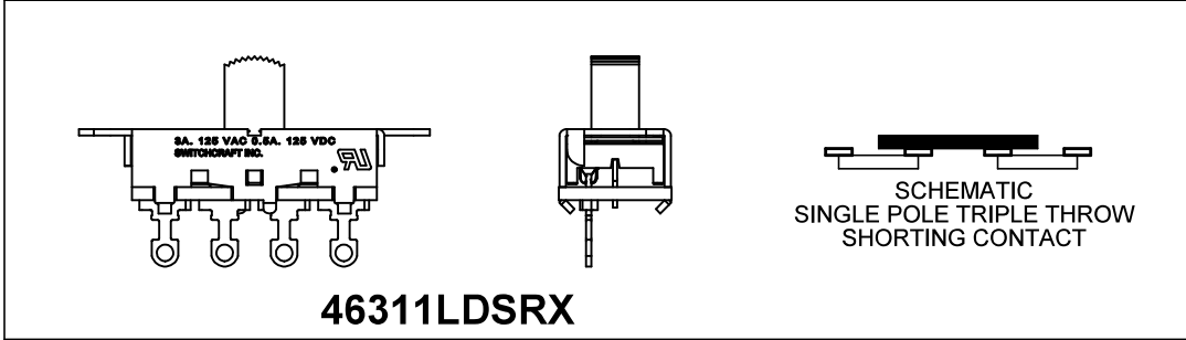
46311LDRX
