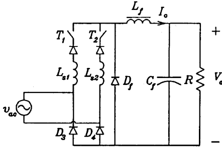
Fig. 5. SRLS voltage rectifier.
