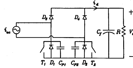
Fig. 6. SRLS current rectifier.
