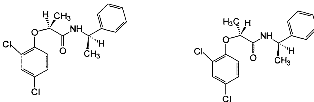
(S)-dichlorprop (R)-phenylethylamine (R)-dichlorprop (R)-phenylethylamine
