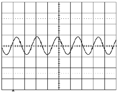
Trace: output voltage (50mV/div.). Time scale: (5 \mu\text{s} /div.).
