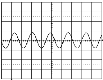
Trace: output voltage (50mV/div.). Time scale: (5 μs/div.).
