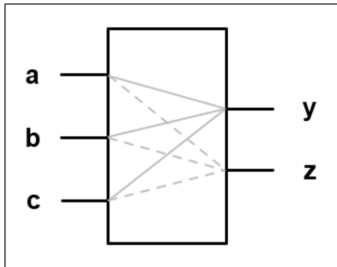
3x2 Crossbar Switch
