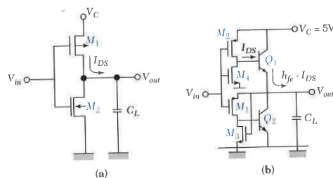
Fig. 31 (a) CMOS logic gate. (b) Bipolar CMOS (BiCMOS) logic gate.
