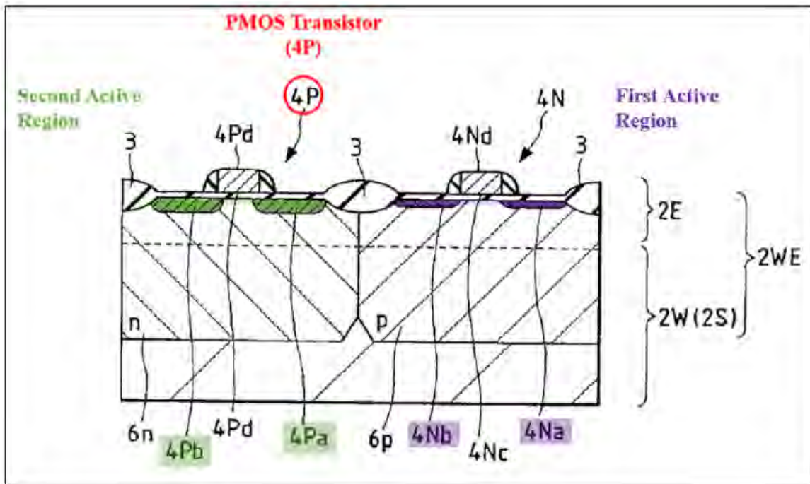
EX1007, FIG. 23.
