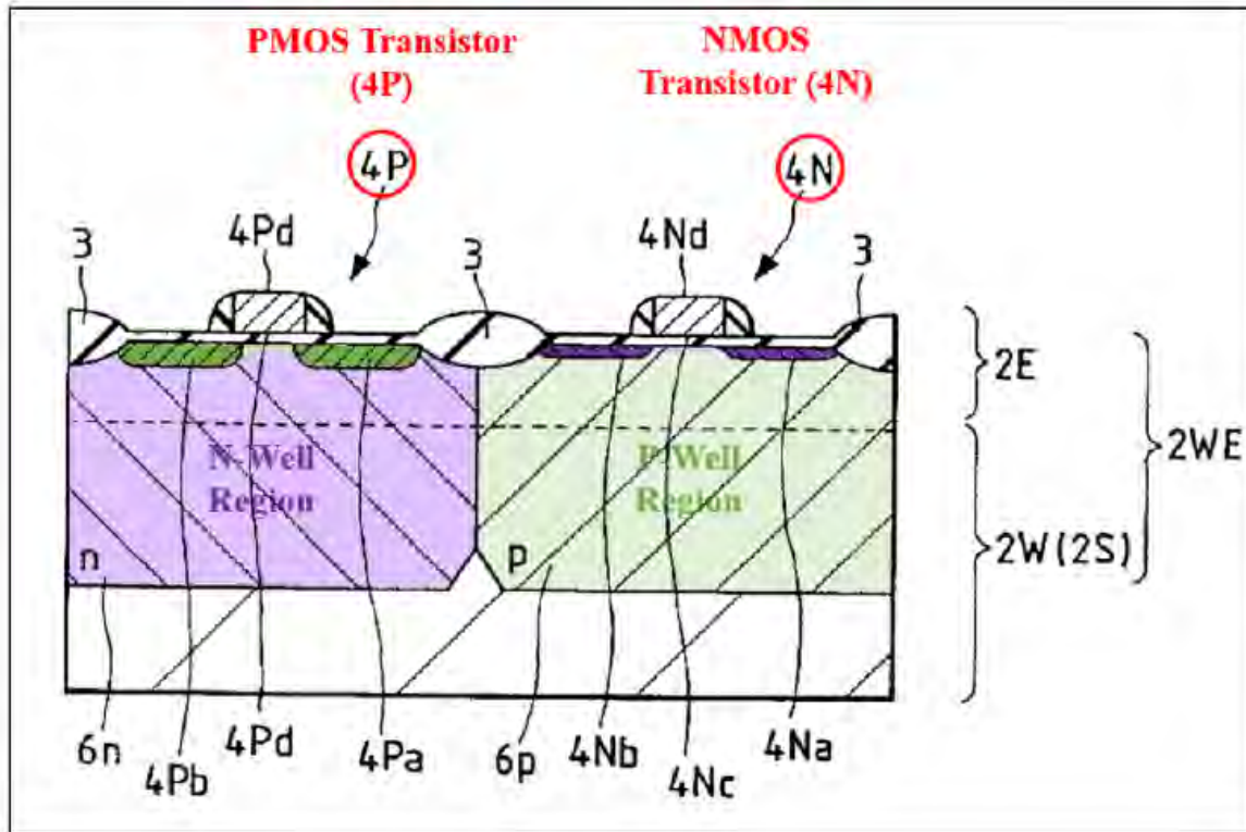
EX1007, FIG. 23.
