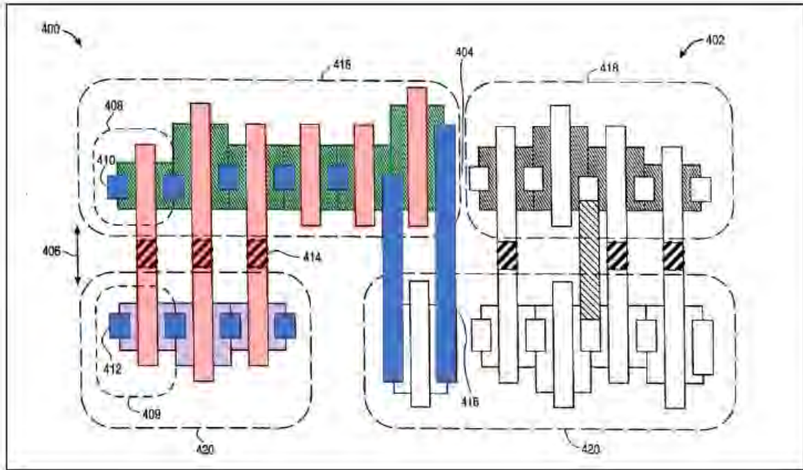
EX1014, FIG. 4.
