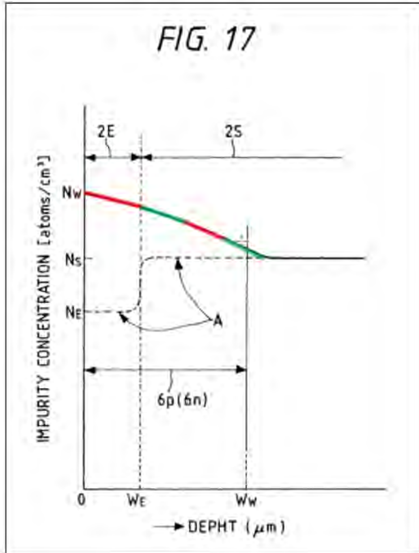
EX1007, FIG. 17.
