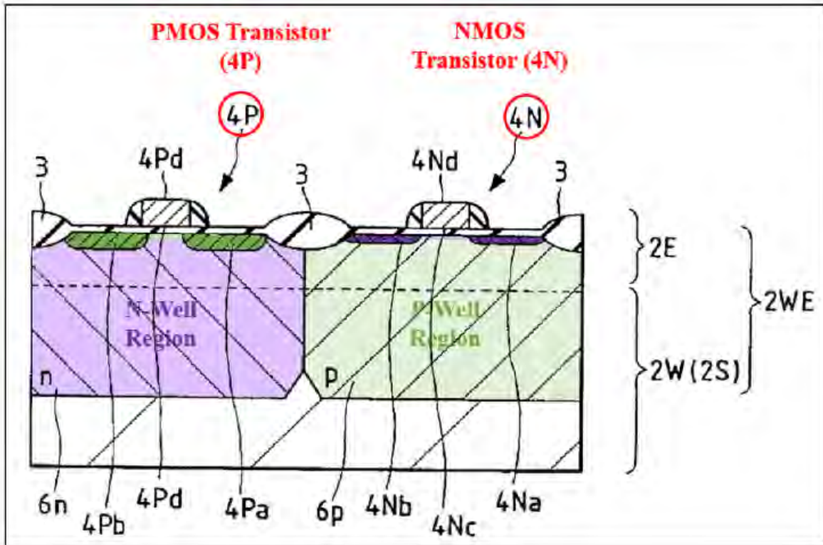
EX1007, FIG. 23.
