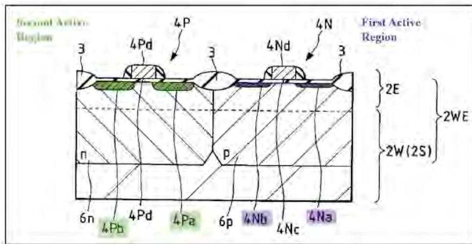
EX1007, FIG. 23.
