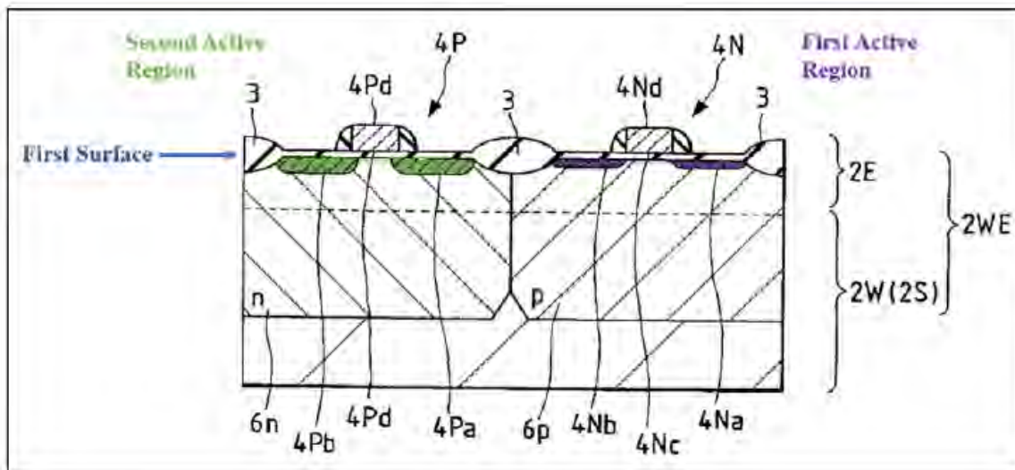
EX1007, FIG. 23.
