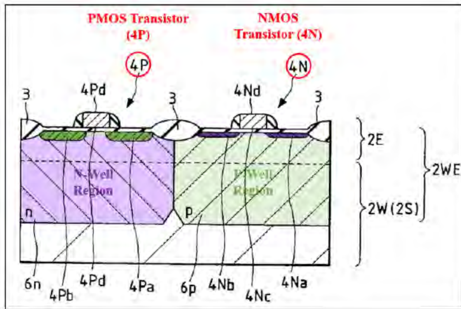
EX1007, FIG. 23.
