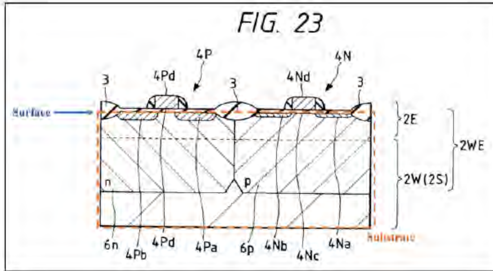
EX1007, FIG. 23.
