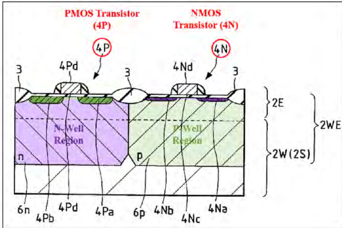
EX1007, FIG. 23.
