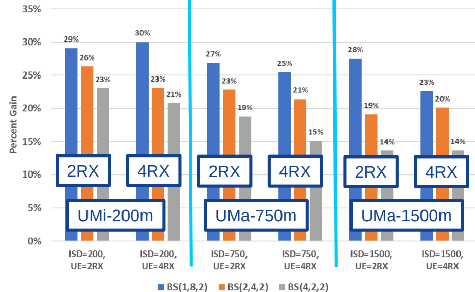
Gain of NR over LTE - Cell Edge SE
