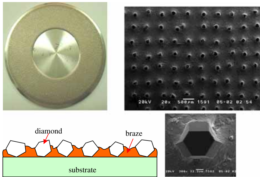
Fig. 1. Brazed diamond disk.
