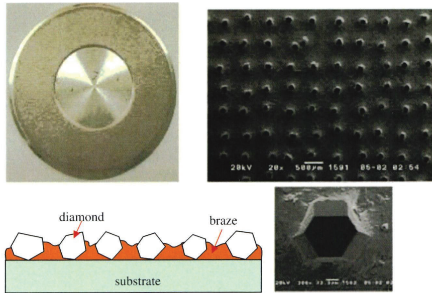
Fig. 1. Brazed diamond disk.
