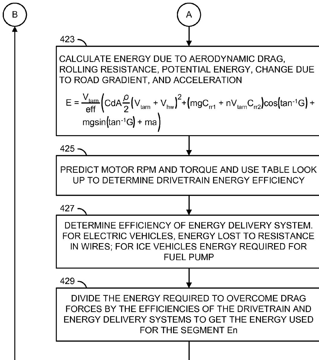
FIG. 4B
