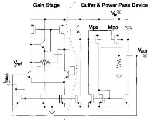
Fig. 9. Low voltage LDO.
