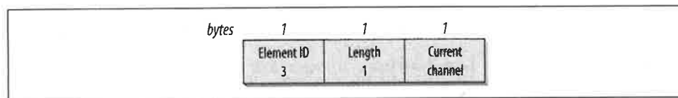
Figure 4-35. DS Parameter Set information element
