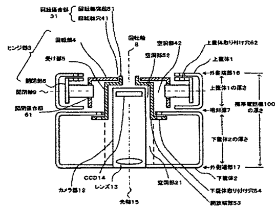
【実施例1】 筐体とヒンジ部とカメラ部の組み立て後の断面図
