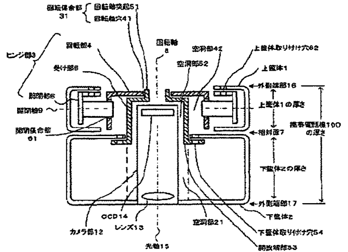
「実例1: 陸体とヒンジ部とカヌラ部の組み立て後の断面図」
