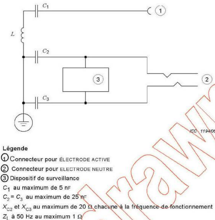
Figure AA.3 – Exemple de circuit PATIENT avec ÉLECTRODE NEUTRE référencée par rapport à la terre aux fréquences de fonctionnement
