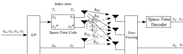
Fig. 4. Hybrid MIMO.
