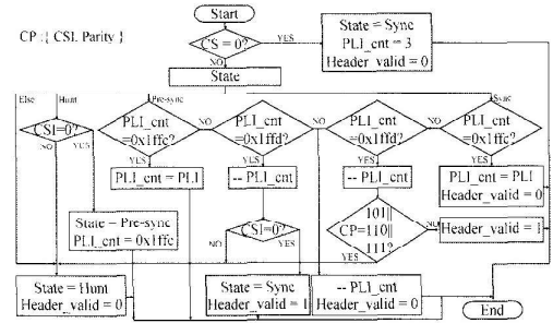
그림 9. 주 상태머신 순서도
