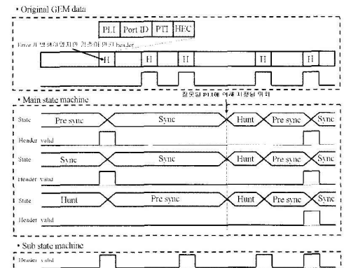
그림 10. GEM 헤더 검출에 실패하는 특수한 경우
