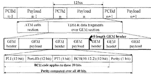
그림 1. G-PON 하향 프레임 구조
