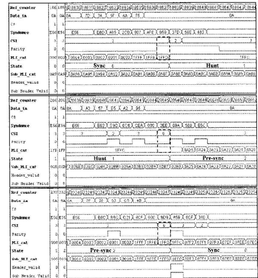
그림 16. 동기손실에서 동기 재획득 과정 Fig. 16. Process of reacquiring synchronization in the loss of synchronization.
