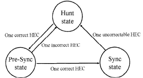
그림 2. GEM 동기 상태머신
