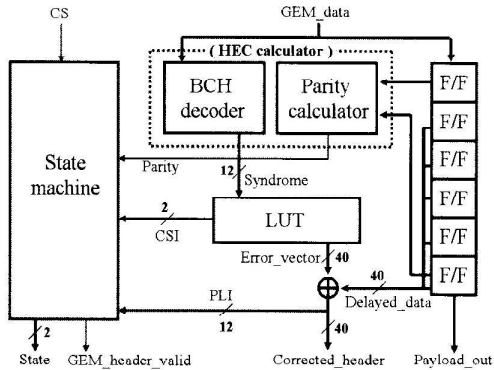
그림 3. GEM 프레임 동기회로도
