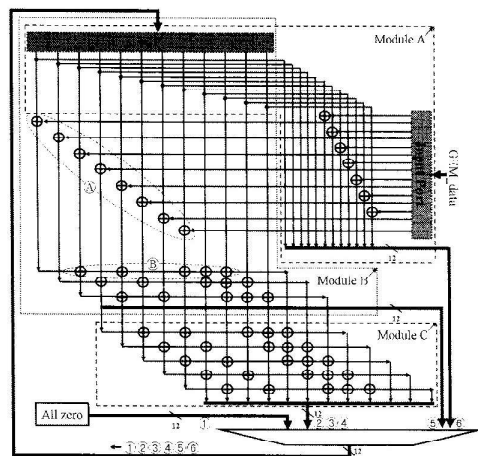
그림 4. BCH 계산기 Fig. 4. BCH calculator.
