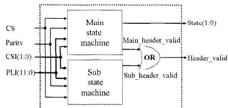
그림 8. 상태머신의 구조
