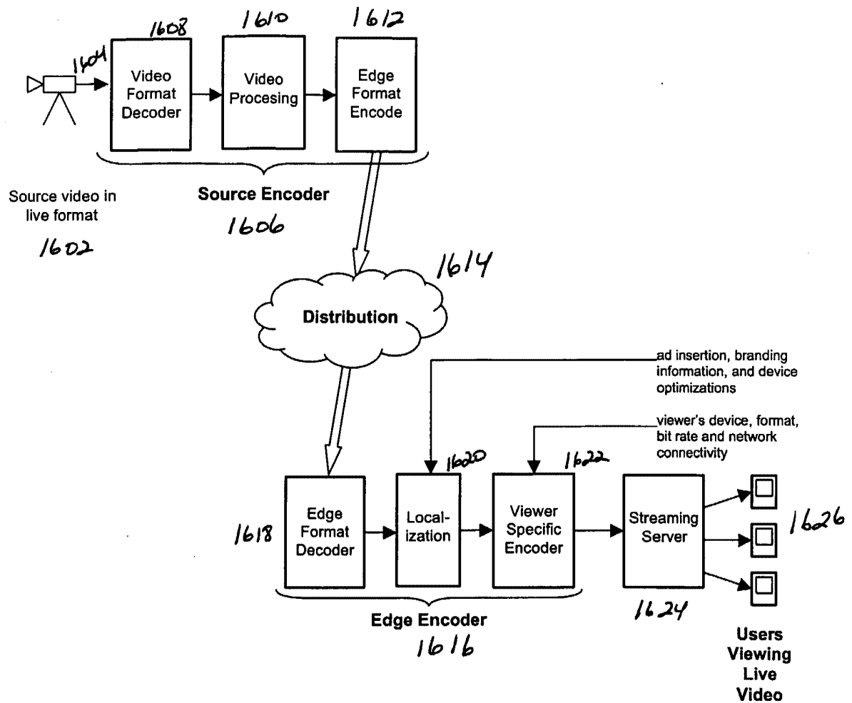
Figure 16 Edge Encoding
