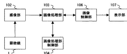
本発明を実施する顕微鏡撮像システムの概略構成を示す図
