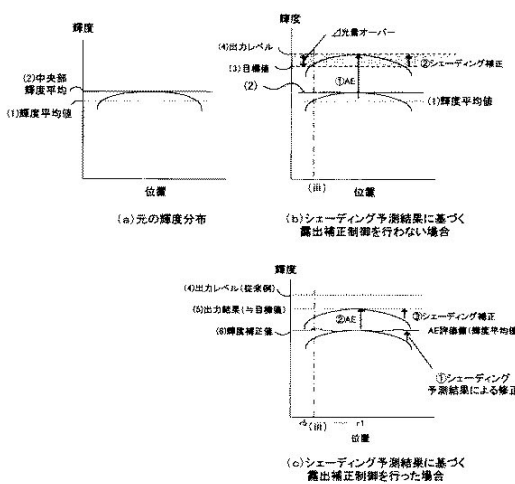
本発明に係るシェーディング予測結果に基づいた露出補正制御の効果を説明する図
