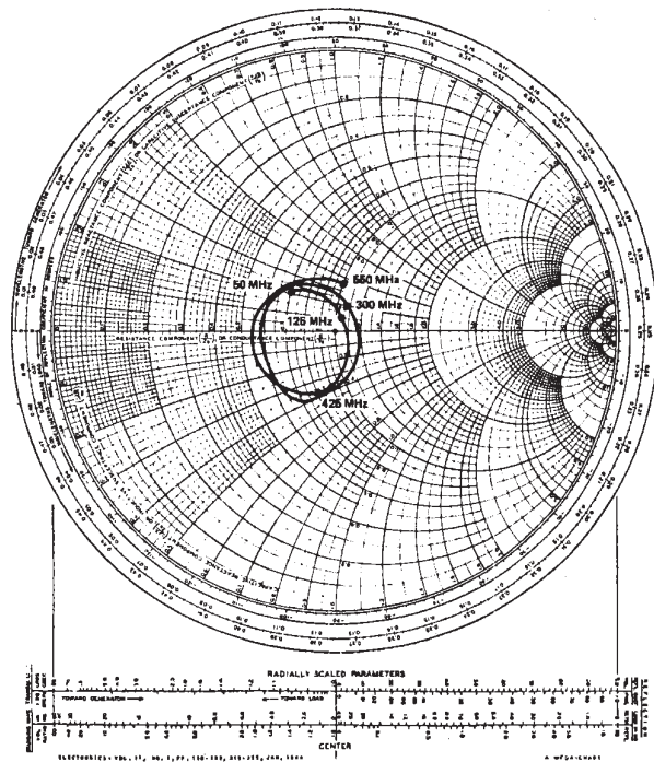
50Ω - 200Ω Balun
