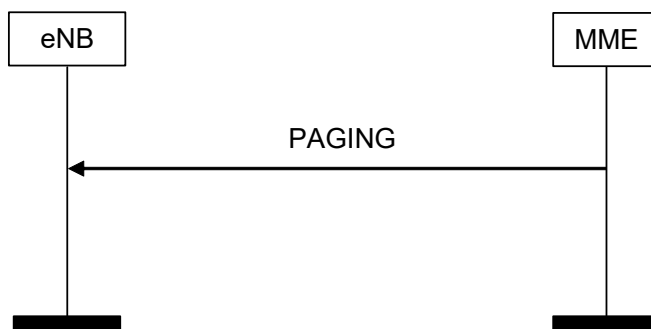
Figure 8.5.2-1: Paging procedure
