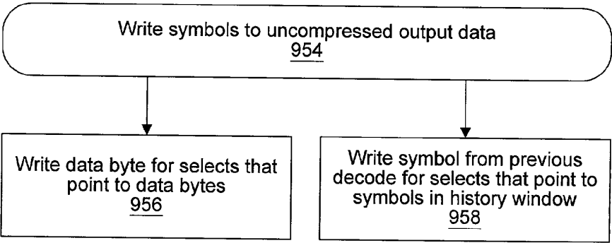
Decompression flowchart Fig. 23e
