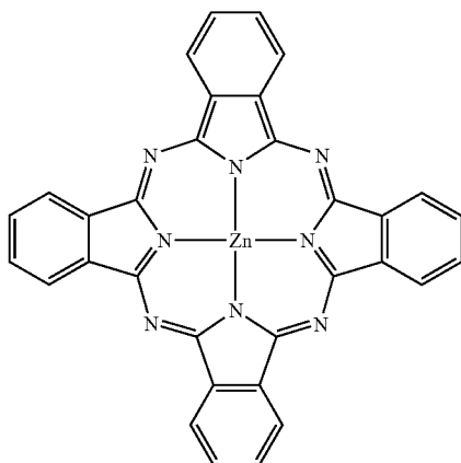
ZnPc
