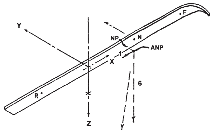
FIG. 10 Test 1.11
