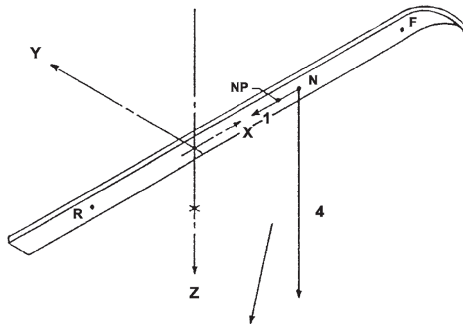
FIG. 13 Test 2.3
