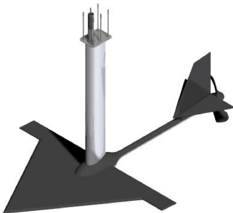
Figur 6 Illustration av Evolos undervattenskropp
