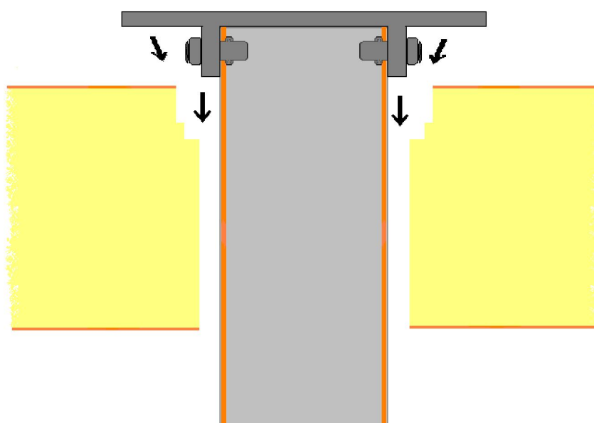
Figur2.infästning steg 1
